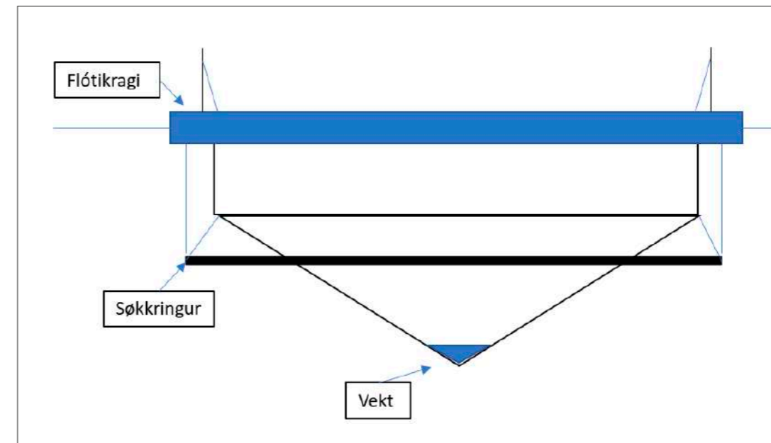
Mynd 2: Ein aliringur við flótikraga, søkkringi og vekt í botninum.
