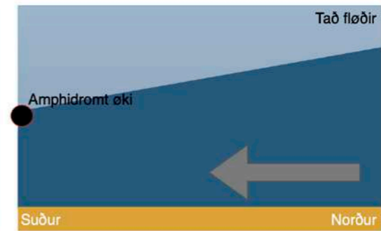
Mynd 5: Einföld lýsing av hvussu rákið kann broytast við sjóvarfallinum nærhendis eitt amphidromt øki.
