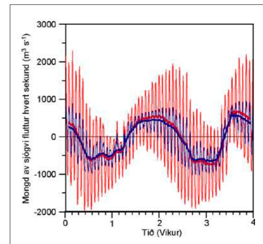
Mynd 8: Mongd av sjógvi flutt yvir Eiðisgrynnuna (reyði liturin), og yvir Streymin (blái liturin). Mongdin er positiv (ovan fyri strikuna), tá sjógvurin ferðast norðureftir. Tunnu strikurnar eru tímavirði. Tjúkku strikurnar eru miðal yvir 25 tímar.
