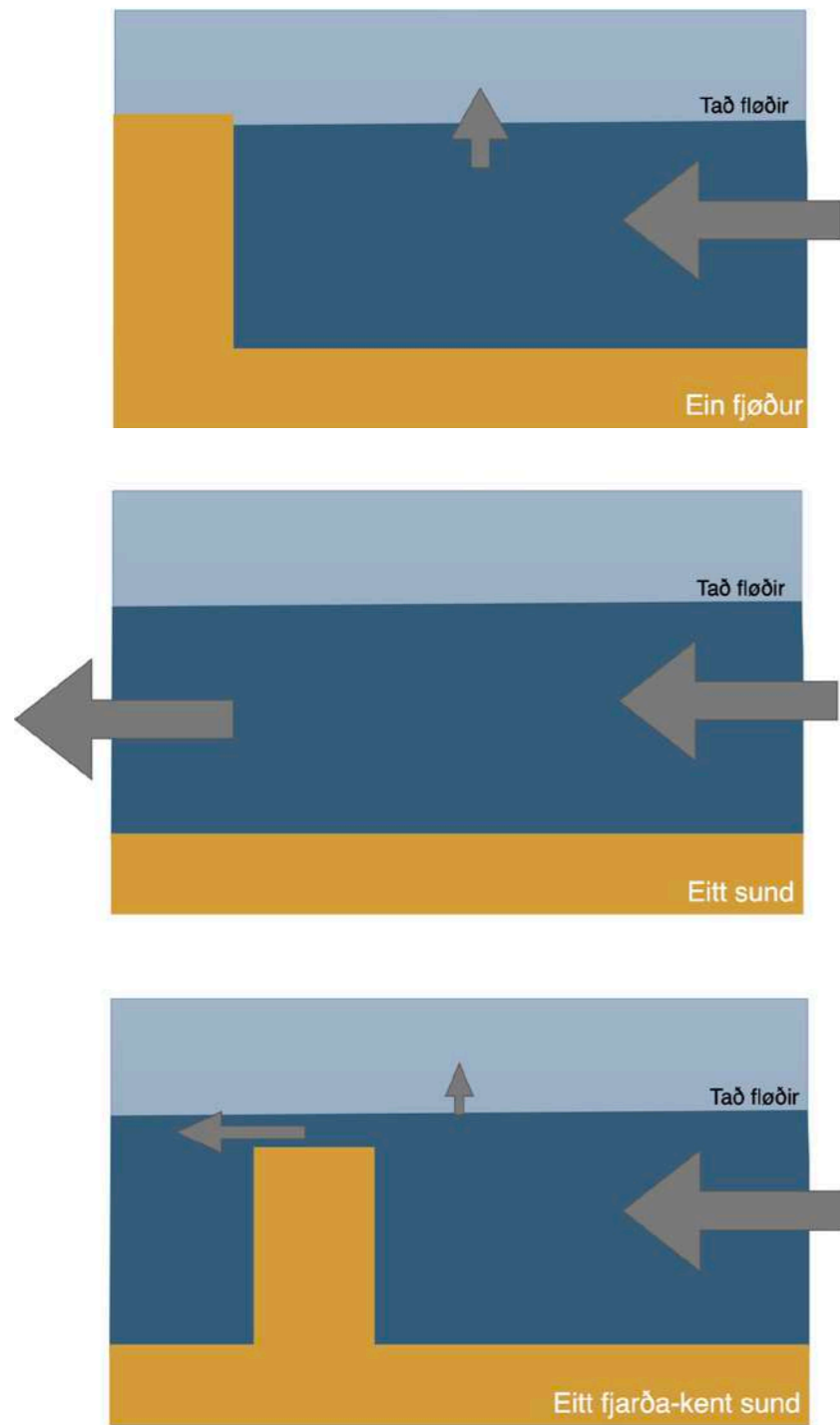
Mynd 6: Lýsing av hvussu sjóvarfallið ávirkar annaðhvørt ein fjørð (ovast), eitt vanligt sund (í miðjuni) ella eitt fjarðakent sund (niðast).
