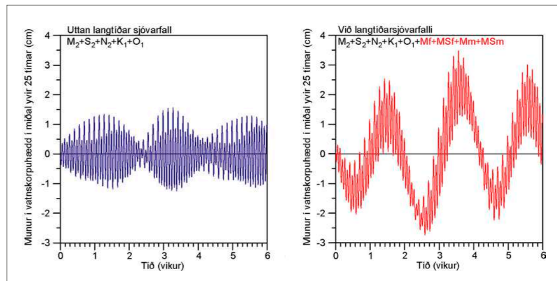
Mynd 9: Munur millum vatnshædd á Eiði og í Tórshavn út frá mátingum hjá Landsverki. Vinstrumegin er bara hálvdagligt og dagligt sjóvarfall. Høgrumegin er langtíðar sjóvarfallið tikið við afturat.
