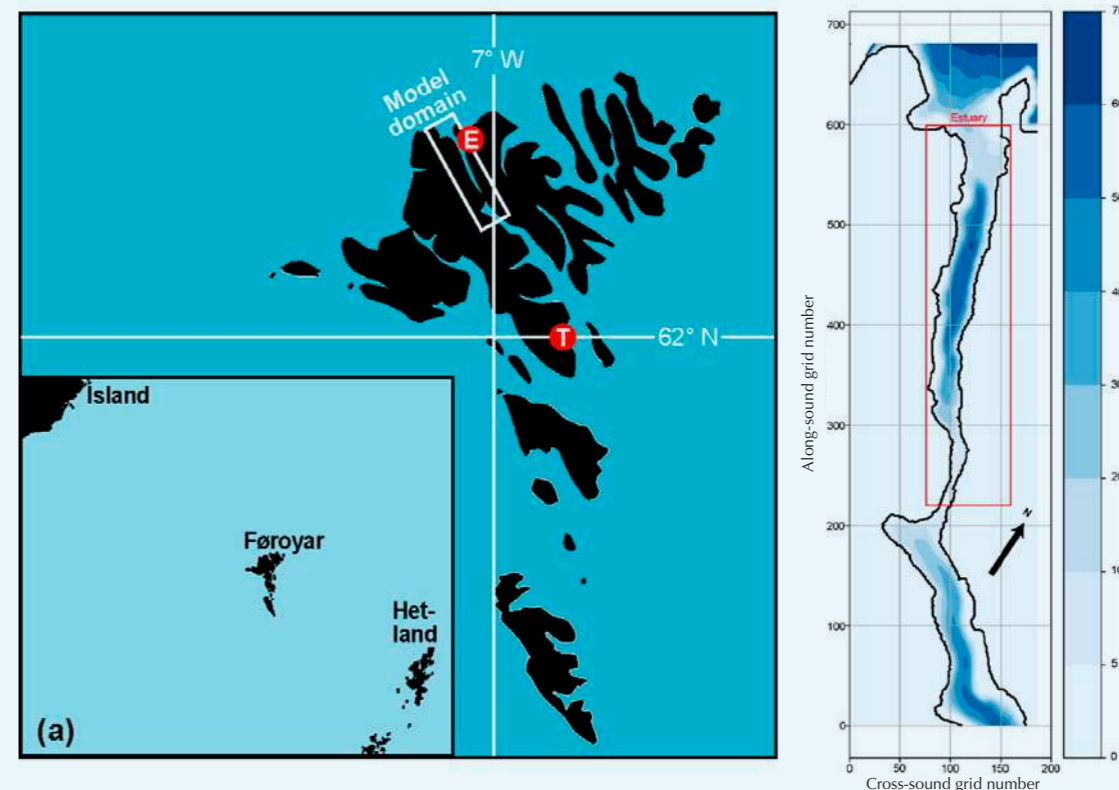
Mynd 2: Til vinstru kort yvir Føroyar. E er Eiði, T er Tórshavn og Model domain er myndlaða økið. Nærmynd av Model domain sæst til høgru.
