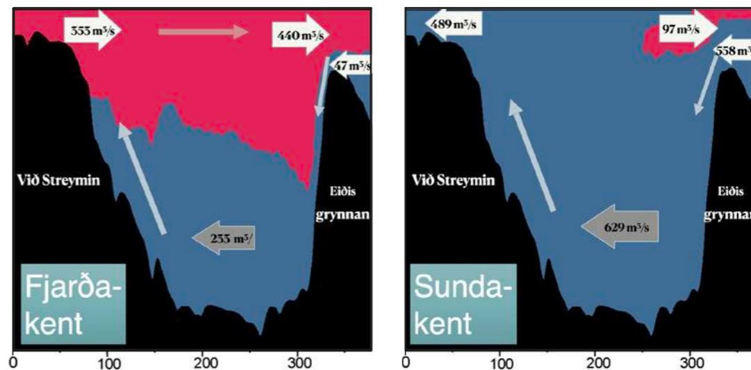
Mynd 3: Rákið av sjógvni tá tað er antin fjarðakent ella sundakent í Sundalagnum norðan fyri Streymin. Reyðu økini vísa norðurgangandi rák. Bláu økini vísa suðurgangandi rák.
